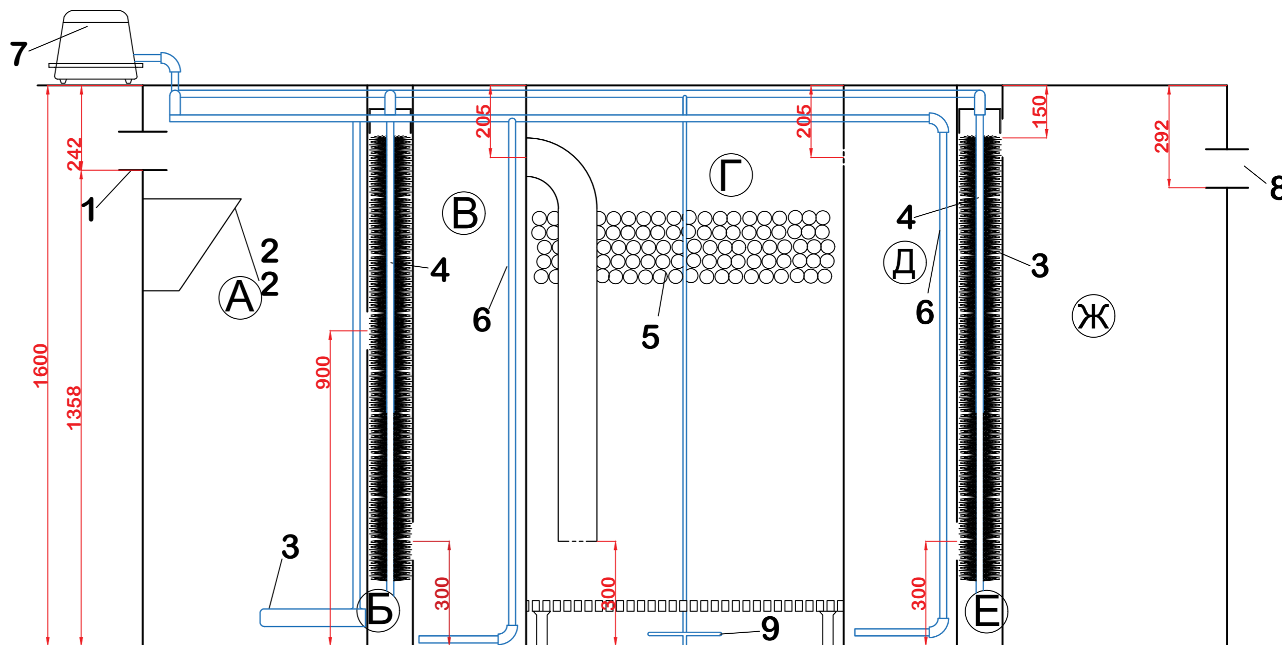
Экспликация зон очистки сточных вод
